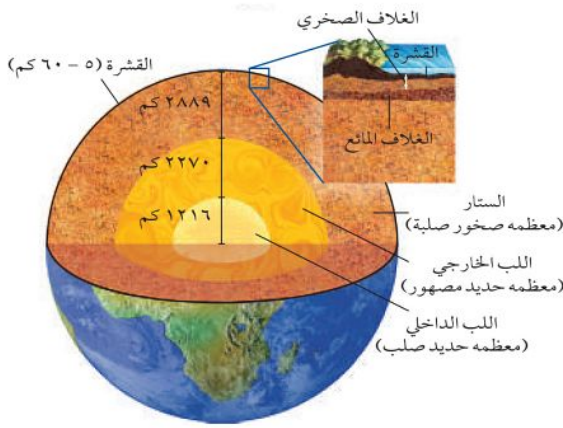
الشكل ١٨ لقد مكّنت الموجات الزلزالية المتولدة من الزلازل العلماء من معرفة تركيب ومكونات باطن الأرض.
